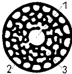
Querschnitt von Amphipora ramosa PH. (10 ×)
