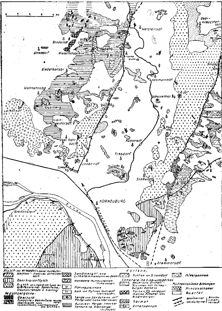
Abb. 3. Karte der Waschbergzone und der Ausläufer des Wienerwald-Flysches N der Donau mit begleitenden Strukturen. — Mit Benützung von Aufnahmen von K. Friedl (Inneralpine Wiener Becken, Wienerwald), Fr. J. Langer (Bisamberg), D. Stur, H. Vettors (Waschbergzone), Bohrergebnissen der Gewerkschaft Austro-gasco (Umgebung von Enzersfeld—Königsbrunn) und der Explora G. m. b. H. und nach eigenen Neubegrehungen (Waschbergzug, Korneburger Becken), zusammen-gestellt von R. Grill.
