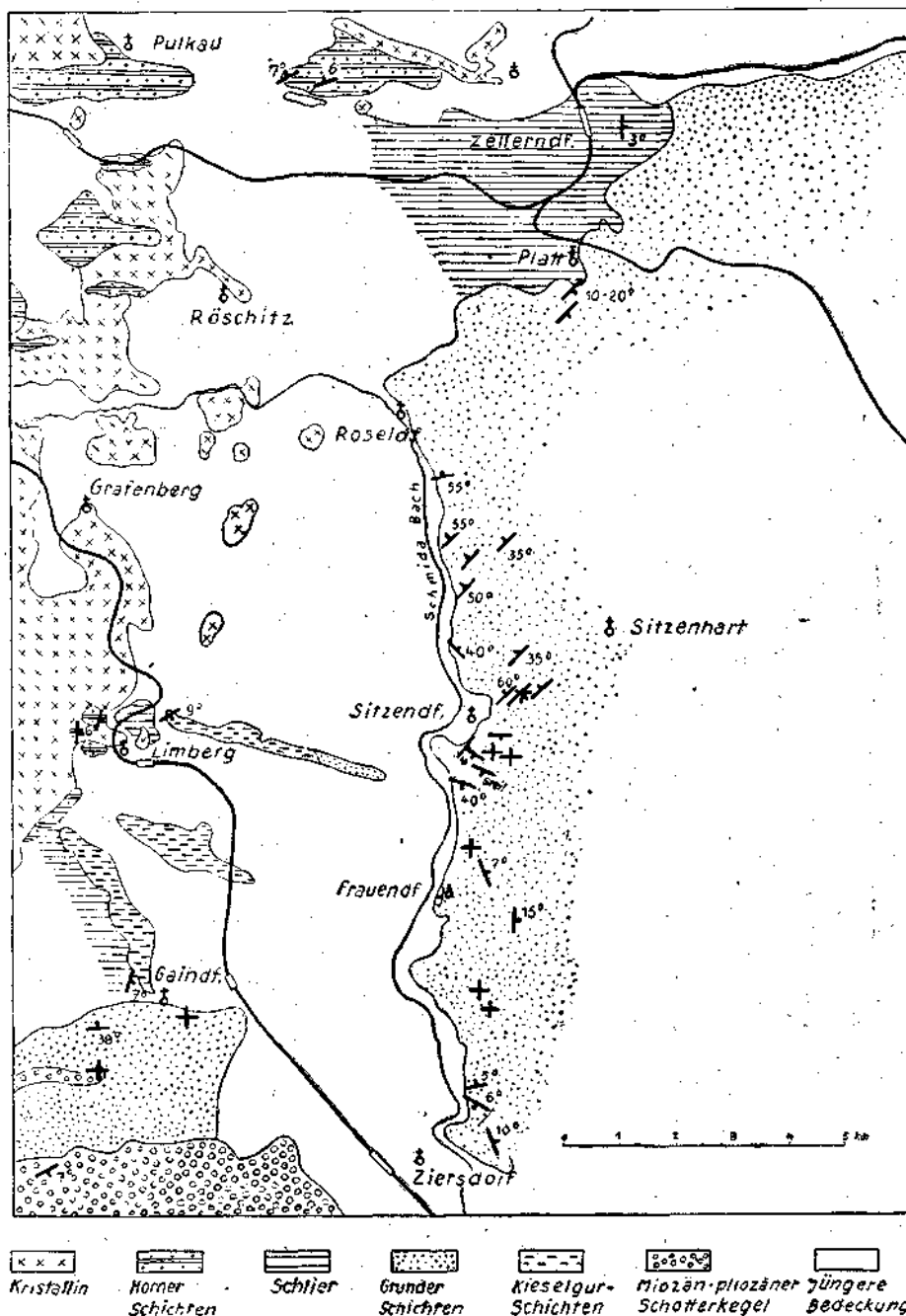
Abb. 2. Skizze der geologischen Verhältnisse in der Umgebung von Sitzendorf—Platt.
