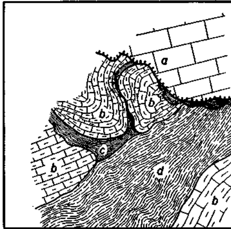
Abb. 2. Eine gefaltete und aufgelinstete Partie der Linse des Blockbergdomes (Lurgrotte). a) Schöckelkalk, b) dunkler, weißgeädertes Kalk, c) Graphitschiefer, d) Tonschiefer (ca. 1:25).
