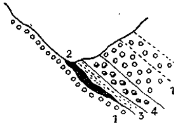
Abb. 4. Detailaufschluß im Wiesergraben. 1. Konglomerat; 2. Glanzkohle; 3. Lettenlage; 4. Sandsteine.
