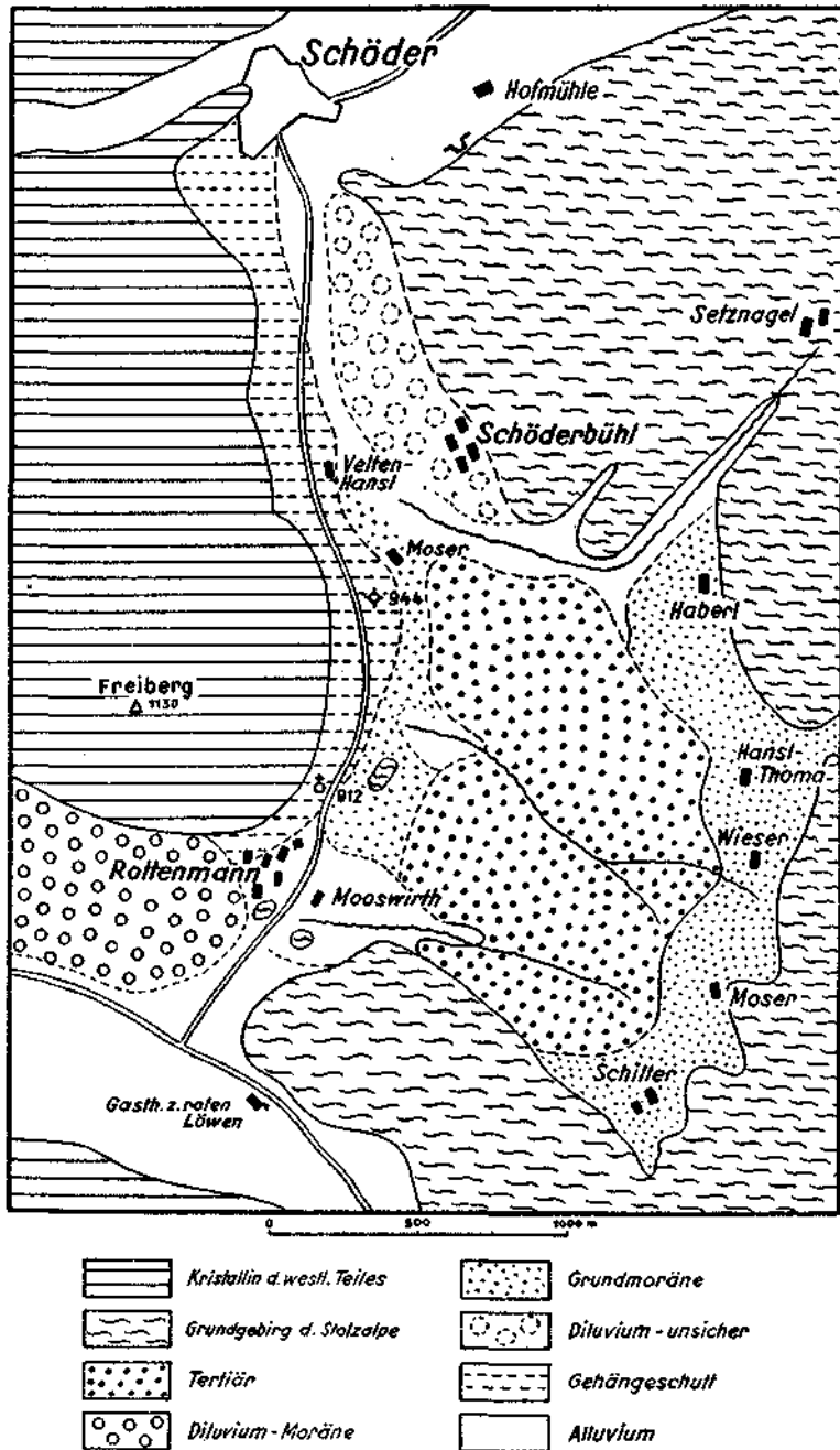
Abb. 1. Übersichtskarte über das Tertiär von Schöder.
