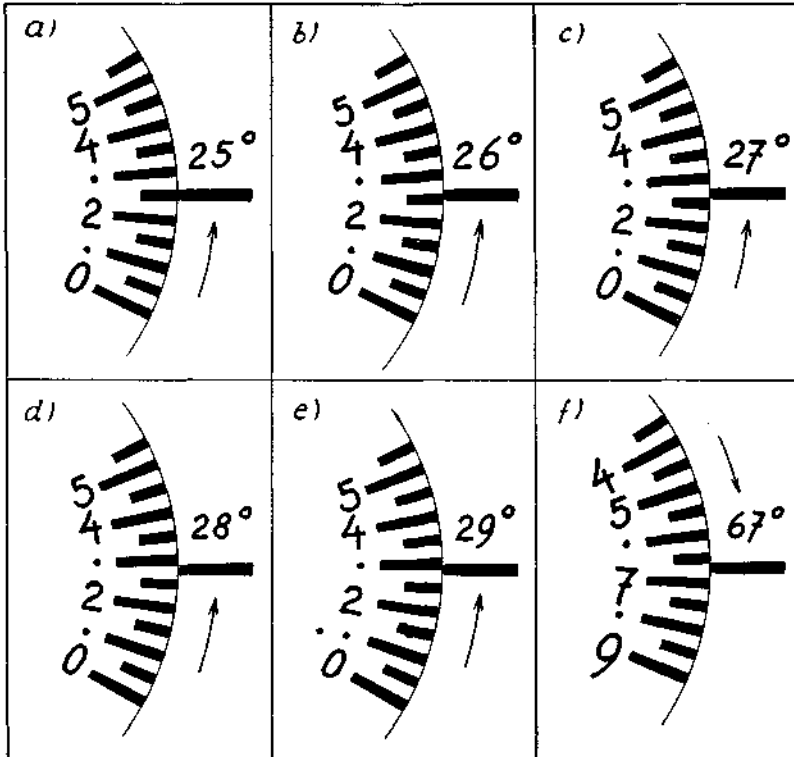
Abb. 3. Beispiel: für die Ablesung von Einzelgraden am Gelenks-Teilkreis. Beispiel a) volle Deckung von Skalenteilstrich und Indexstrich, daher Ablesung gemäß der Bezeichnung des Skalenteilstriches; Beispiele b) und e) halbe Deckung, daher 1^\circ Abweichung gegenüber dem Teilstrich; Beispiele c), d) und f) Randberührung zwischen Skalenteilstrich und Indexstrich, daher 2^\circ Abweichung gegenüber dem Teilstrich; Hierbei Richtungssinn der Skalenteilung beachten! (Pfeile der Abbildung); a) bis e) entspricht der roten, f) der schwarzen Teilung am Kompaß.
