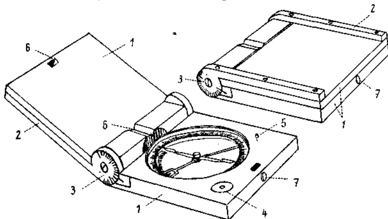
Abb. 1. Skizzen des beschriebenen Kompasses mit geöffnetem und geschlossenem Gehäusedeckel. 1. Holzgehäuse mit Bussole üblicher Ausstattung. 2. Metall-Anlegeleisten am Deckel. 3. Vertikal-Teilkreis im Deckelgelenk mit Ableseindex. 4. Dosenlibelle. 5. Arretierstift der Bussolenadel. 6. Visierbeilفة. 7. Verschluss. Abmessungen des Kompasses: 9,5 \times 11,5 \times 3 cm.
