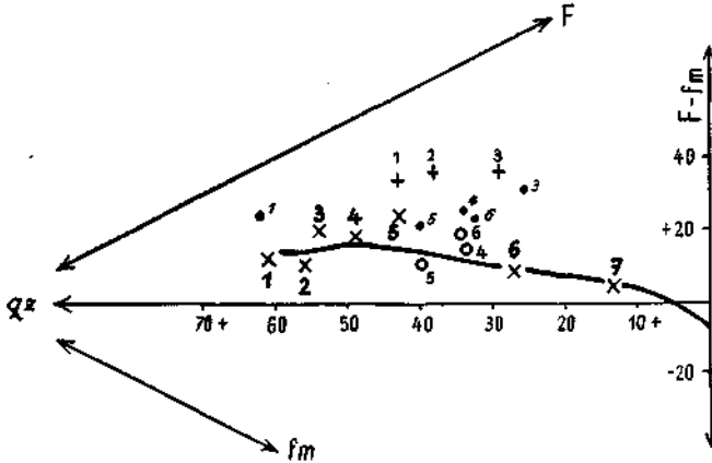
Abb. 1. Ausgezogene Kurve = Lage der Projektionspole (mit × bezeichnet) der „normalen Tiefengesteine“ des Waldviertels. 1 = Granite Typus Eisgarn, 2, 3 = Granite Typus Mauthausen, 4 = Granodiorit von Maria Schnee, 5 = Granit Typus Weinsberg, 6 = Quarzdiorit von Gebharts, 7 = Opdalit von Dornach. 1—6 (mit × bezeichnet) sind die Projektionspole der in der Arbeit erwähnten Gesteine (Nr. 2, Amphibolit ist weggelassen); davon 4—6 (mit ° bezeichnet) nach Verrechnung von Titanit. Zum Vergleich: 1 (mit + bezeichnet) ist Granit(gneis) Wolfshof, 2 und 3 sind Mischgesteine von Landshaag.
