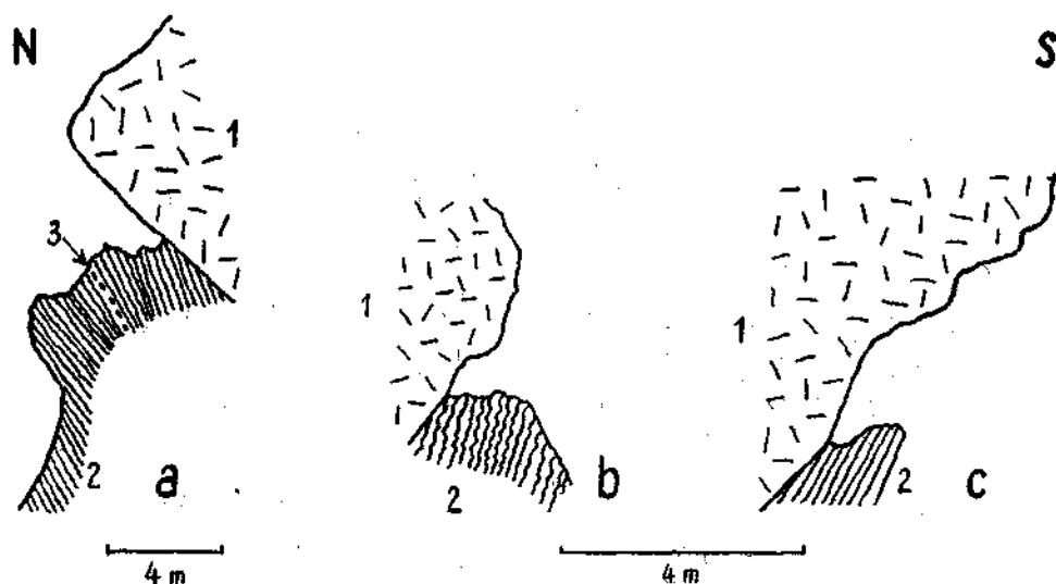
Abb. 2. Die Überschiebung des Hauptdolomits auf das Cenoman. 1 = Hauptdolomit; 2 = Cenoman; 3 = Lage mit Hornsteinkauern.
