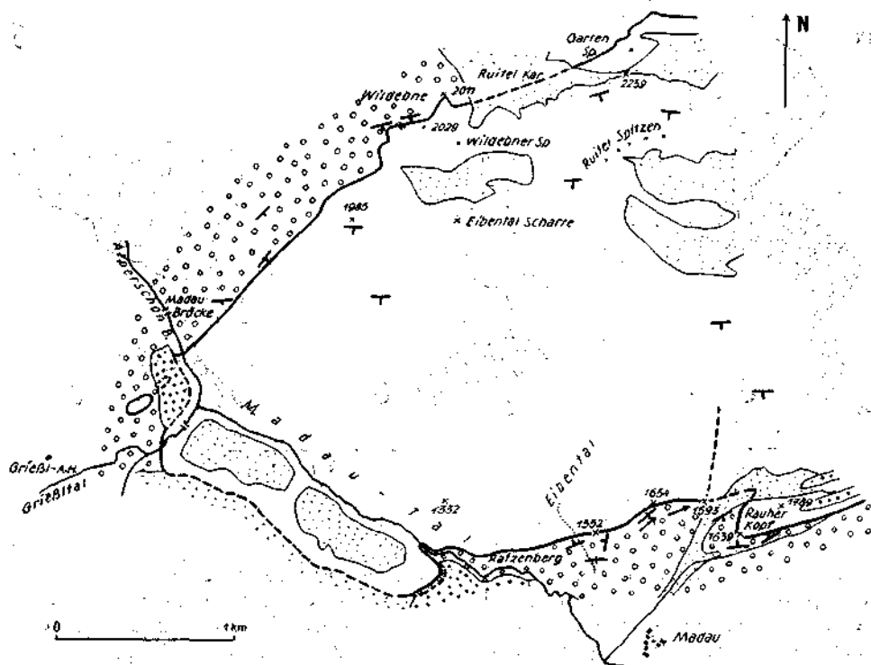
Abb. 1. Die Ruitelspitzen. Gezeichnet auf Grundlage der Karte 1:25.000, Blatt Parseierspitz-Gruppe von O. AMPFERER.
