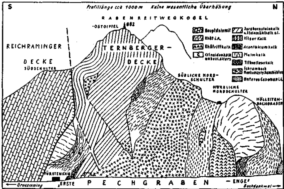
Abb. 2. Profil Reichraminger/Ternberger Decke über das Ostende des Schiefersteinzuges, den Ostabfall des Rabenreitwegkogels (Rabenreitwegkogel-O-Gipfels) an der Westseite der ersten Pechgraben-Enge“ bei Großraming (Oberösterreich). — Unter Benützung der Darstellungen von GEYER auf Blatt Weyer der K. k. Geol. R.-A., Wien 1912, und LOGTERS auf dessen Geologischer Karte der Weyerer Bögen zwischen Laussatal und Pechgraben, in: „Zur Geologie der Weyerer Bögen etc.“, Jahrb. Oberöterr. Musealverein, 87. Bd., Linz 1937, S. 369, sowie der bezüglichen im Lit.-Verzeichnis zu vorliegender Arbeit angegebenen und der durch dasselbe gedeckten Literatur.
