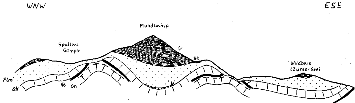
Abb. 4. Schematisiertes Profil durch präjurassisch angelegte Sättel zwischen Spullersgümpel und Zürser See; ON = Oberrorische Kalke; Kö = Kösener Schichten; OK = Oberrhätkalk; LI = roter Unterlias-Kalk; Flm = Fleckenmergel; SK = Schwellenkalke; Kr = Kreideschiefer.
