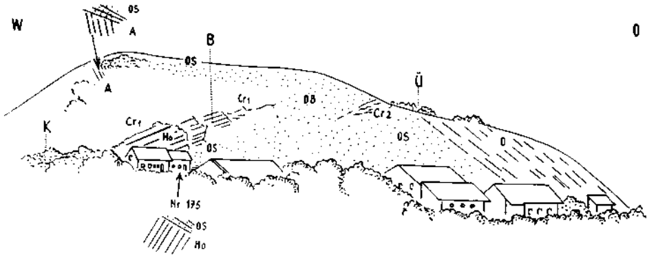
Abb. 4. Blick zur Ölberg S-Seite. Die Skizze soll die diskordante Auflagerung des Cenomans (OS, DB) über die verschiedenen jurassisch-neokomen Schichtglieder (A, K, Cr, Ho) des gegen N überkippten S-Flügels der Ölbergmulde und die Überschiebung der Dolomitscholle (O) veranschaulichen.
