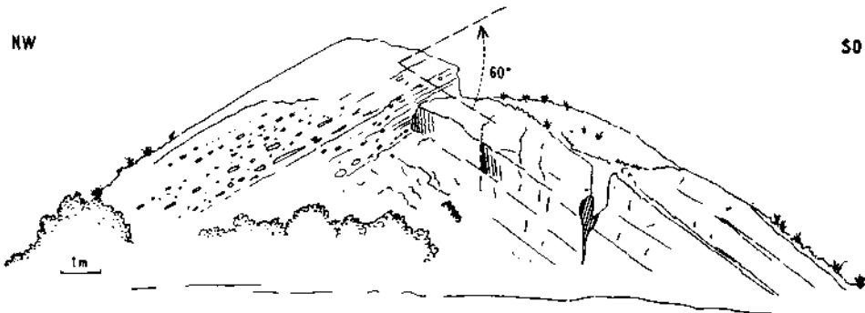
Abb. 1. Aufschluß NO Alland Nr. 141, S des Friedhofes: 30^\circ NW-fallendes Gosaugrundkonglomerat in 60^\circ iger Winkeldiskordanz zum liegenden, 30^\circ SO-fallenden, hellen Mitteltriaskalk der Ötscherdecke. Im Kalk befindet sich eine mit Pisolith-führenden Bauxit erfüllte Kluft. Der Bauxit stellt gewiß den Rest einer mit der Gosautransgression vom Festland her eingeschwemmten Ablagerung dar.
