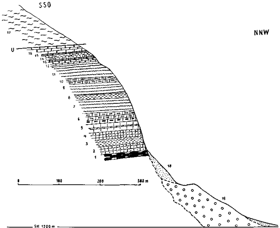
Abb. 1. Profil durch den Mulischrofen.
