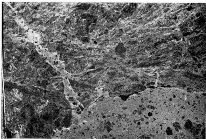
Ungestörter Intrusivkontakt von Quarzdioritporphyr mit Mylonit der Donaustörung. Dünnschliff in Dunkelfeldbeleuchtung, ca. 3,5fach vergrößert. (Photo THIELE.)
