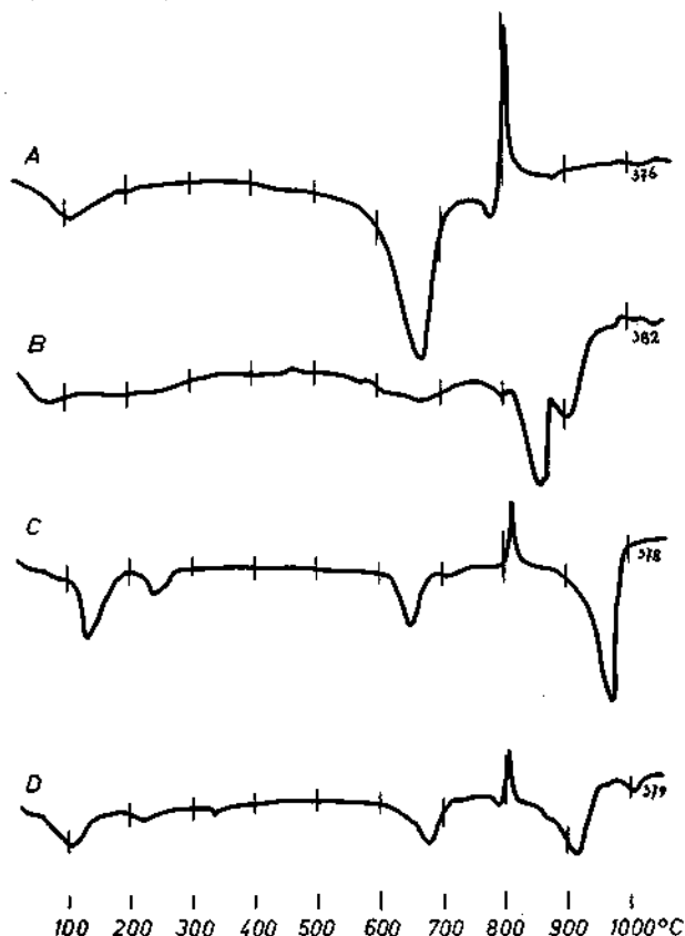
Abb. 1. DTA-Kurven von Chrysotil und Ophicalcit vom Steinbruch Tommach bei Gstadt
