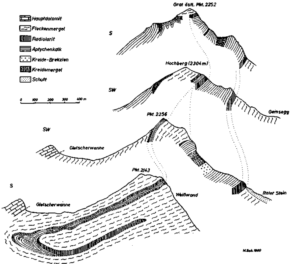
Abb. 3. Kulissenprofil durch die Hochberg-Mulde
