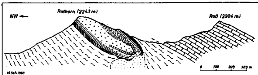
Abb. 4. Ansichtsprofil der Rothorn-Mulde, vom Feuerstein aus gesehen. Signaturen wie Abb. 3.
