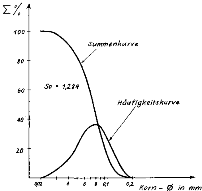
Abb. 1. Korngrößen-Verteilung von 100 Pseudooideen. Zlambach-Mergel des Rohrmoos. Schliff R 4.
