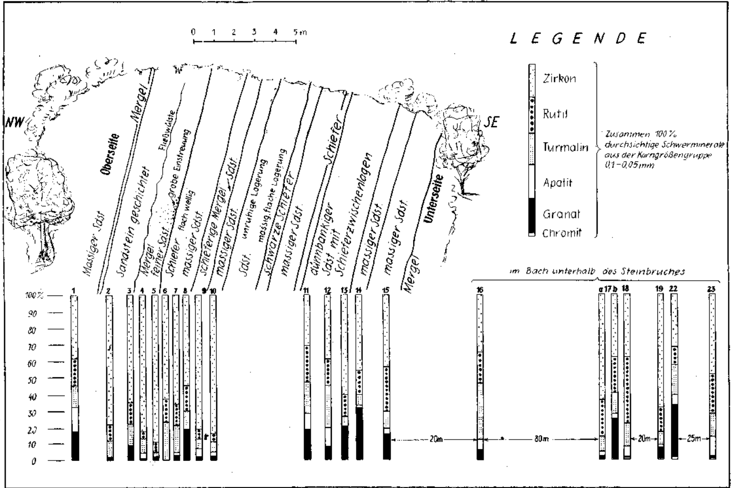
Abb. 1. Steinbruch NW Hois, SE St. Corona.
