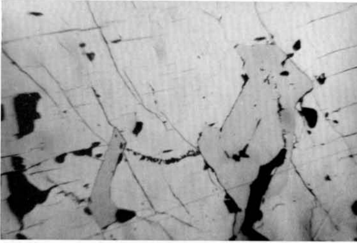
Abb. 2. Magnetit mit Ilmeniteinschlüssen, 250mal, Ölimmersion.
