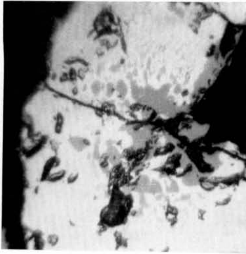
Abb. 4. Magnetit mit Verdrängung von Maghemit, 600mal, Ölimmersion.
