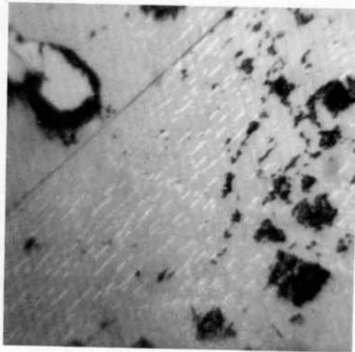
Abb. 5. Ilmenit mit Entmischungen von Hämatit, 600mal, Ölimmersion.
