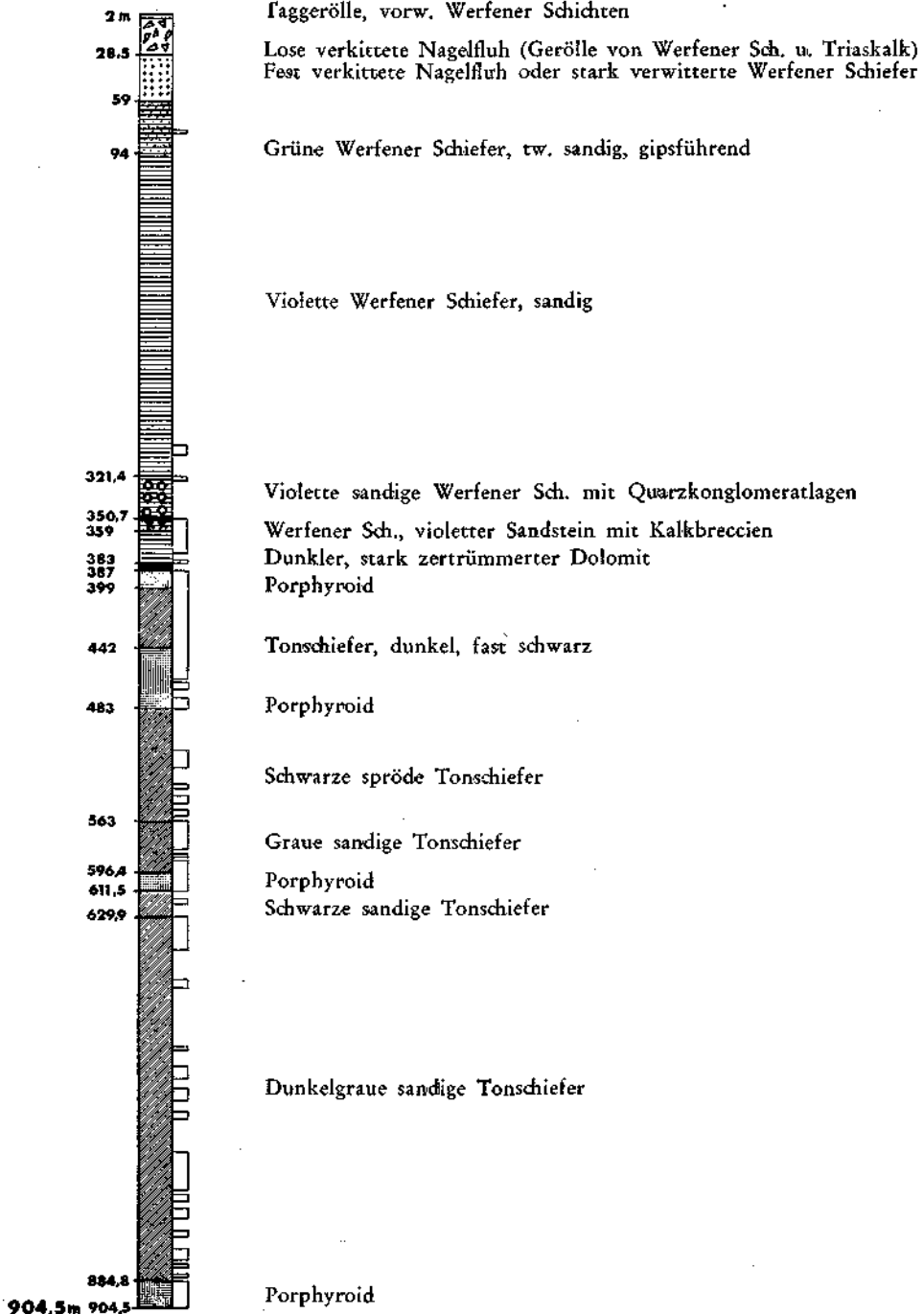
Abb. 1: Profil der Tiefbohrung Geieregg I bei Eisenerz
