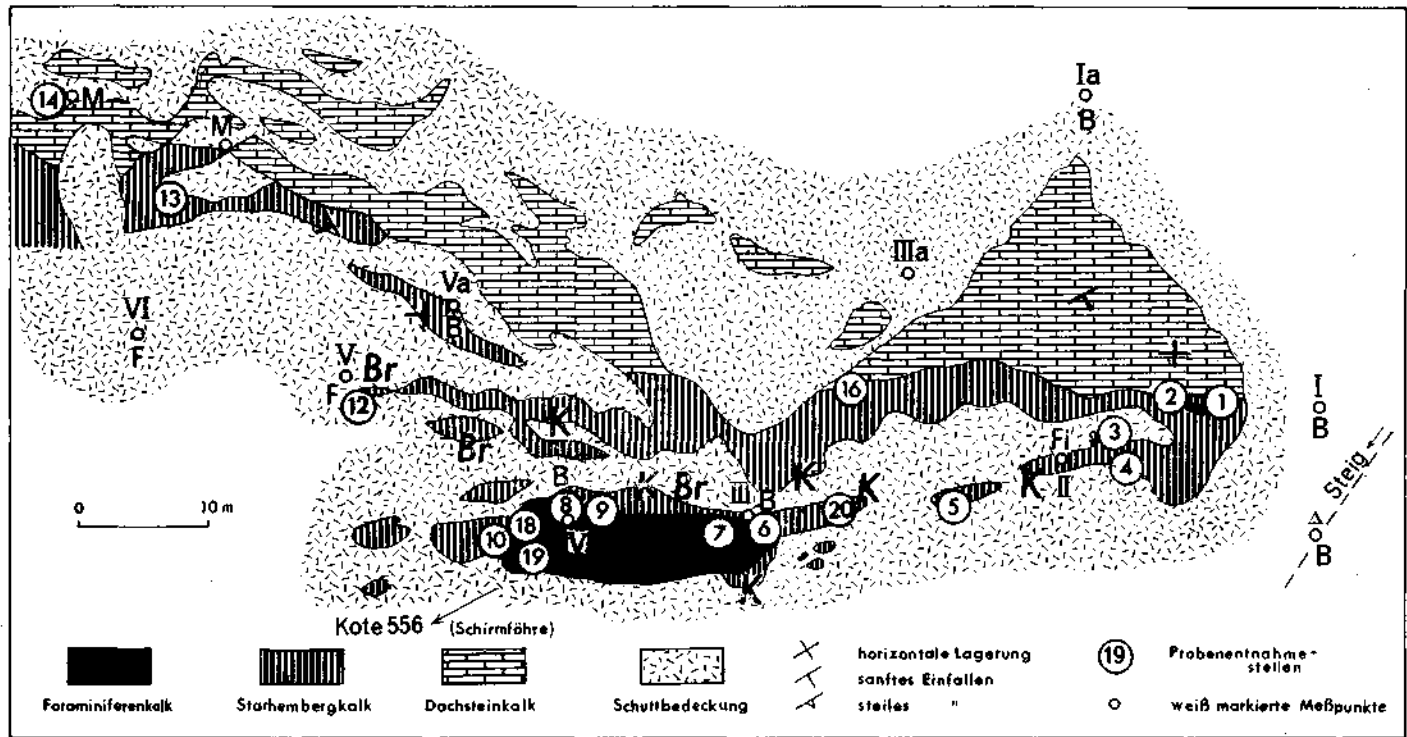
Abb. 2. Geologische Kartenskizze
