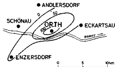
Abb. 6 KALKBRECCIE MÄCHTIGKEIT
