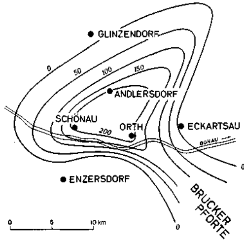
Abb. 5 ORTHER KONGLOMERAT MÄCHTIGKEIT
