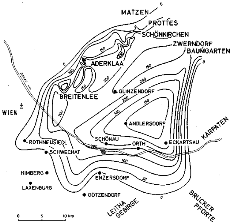
Abb. 4 ADERKLAER KONGLOMERAT MÄCHTIGKEIT
