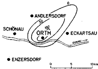
Abb. 5 ORTHER KONGLOMERAT MÄCHTIGKEIT
