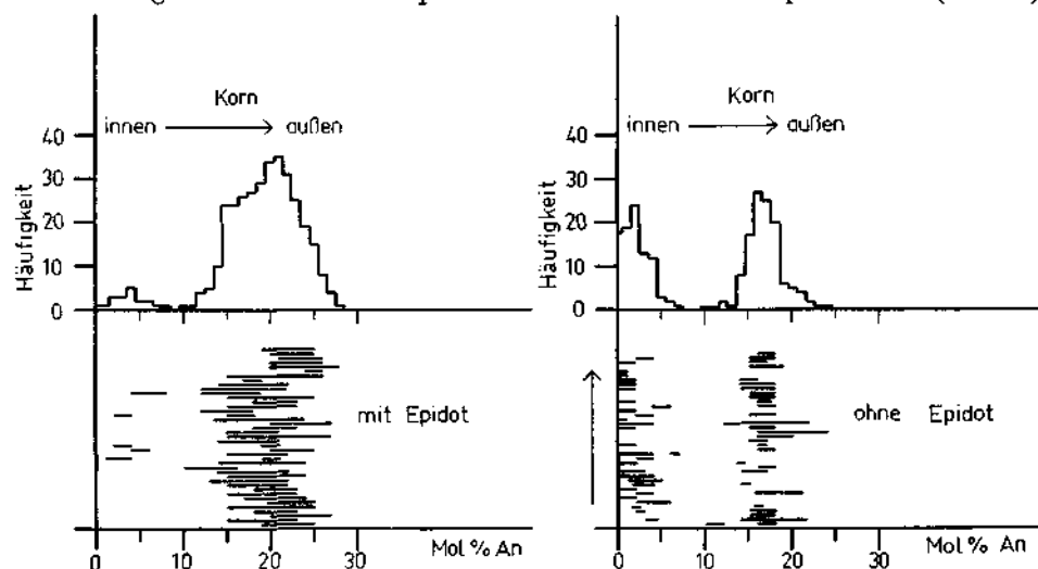
Abb. 4. Variation der Anorthit-Gehalte inverszonarer Plagioklase Plag II von 41 Paragenesen mit Epidot und 40 Paragenesen ohne Epidot.
