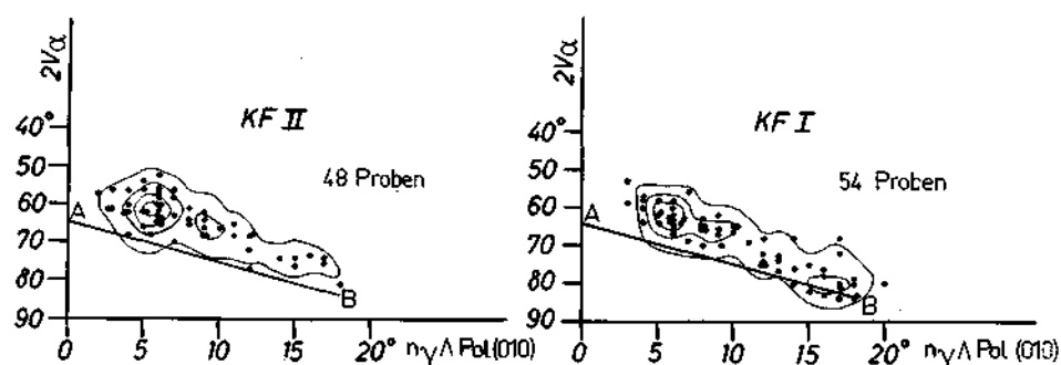
Abb. 6: Beziehung zwischen optischen Achsenwinkel 2V_{\alpha} und Auslöschungsschiefe n_{\gamma} \Delta \text{Pol (010)} der Kalifeldspäte. A—B: "stable microcline line" nach F. Laves et al. 1967. Zur Darstellung kamen die Extremwerte der Proben.
