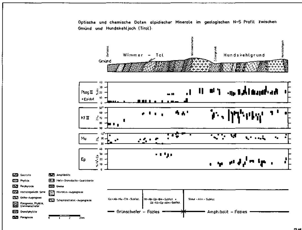
Abb. 3. Optische und chemische Daten alpidischer Minerale im N-S Profil zwischen Gmünd und Hundskehljoch (Tirol).
