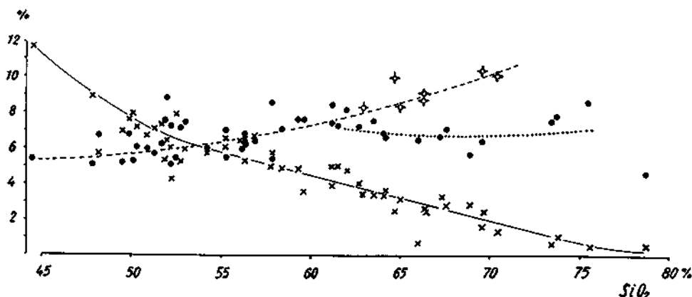
Abb. 8. Variationsdiagramm der nicht alkalischen Ganggesteine aus der Böhmischo-Mährischen Anhöhe und aus dem niederösterreichischen Waldviertel (Gewichtsprozent). \times - \text{CaO} , \bullet - \text{Na}_2\text{O} + \text{K}_2\text{O} ( \diamond - saure Ganggesteine aus der Umgebung von Persenbeug). Der Peacock Index gleicht 54.
