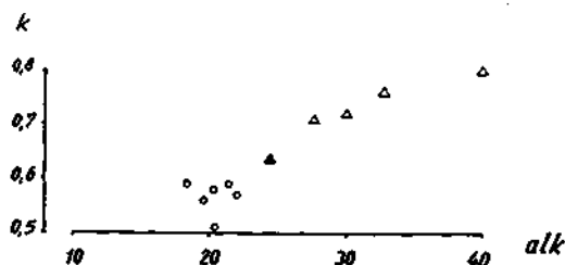
Abb. 5. alk-k-Diagramm der Ganggesteine aus der Umgebung von Raabs. \circ - Pyroxen-Granodioritporphyrite und Mikrosyenite, \blacktriangle - Alkalimikrosyenit, \triangle - Alkalimikrogranite.
