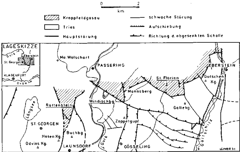
Abb. 1. Tektonische Übersichtsskizze.
