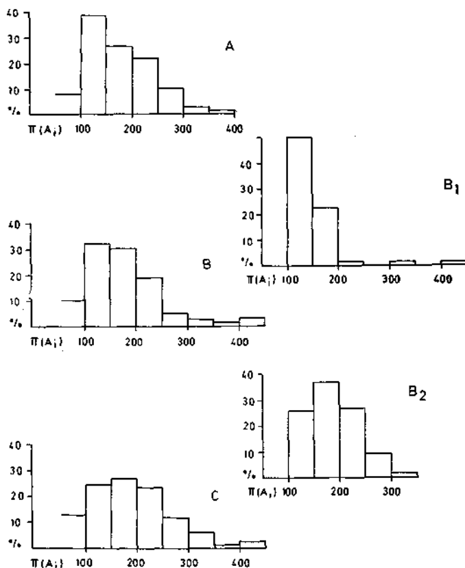
Abb. 5. Morphogramme der Abplattungsindizes für die Schichten A, B, C, B 1 nur kantengerundete, B 2 nur gerundete Gerölle aus Schicht B.
