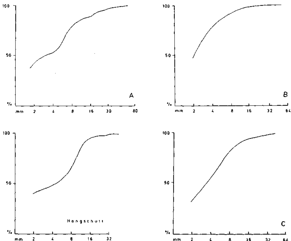
Abb. 4. Kornsummenkurven der Schichten, A, B, C, sowie von rezentem Hauptdolomithangschutt.
