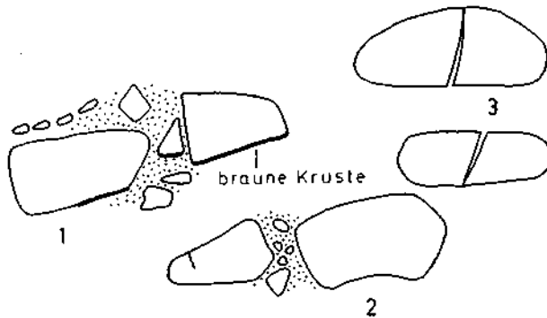
Abb. 3. Kalottenförmige Gerölle aus Schicht B (natürliche Größe).
