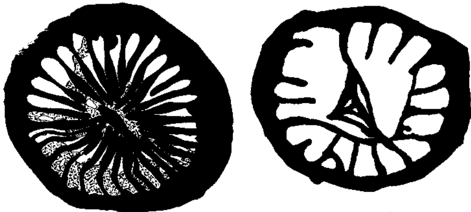
Abb. 20. Sinophyllum sp., Productus -Limestone, Loc. T 67—88, River 1 (MMH 11938). 3,6 ×. Abb. 21. Leonardophyllum ? sp., Productus -Limestone, Loc. 1-Pl. (MMH 11939). 10 ×.
