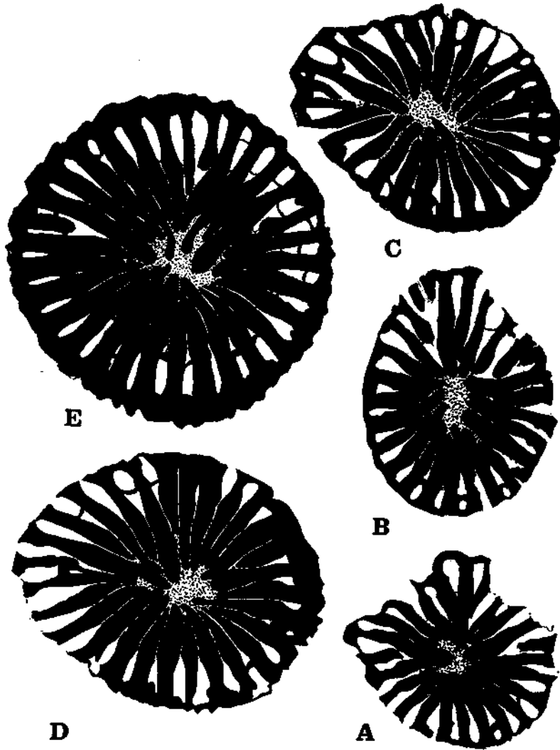
Abb. 13. Lytvolasma (?) cf. geinitzi (TOULA, 1875), Productus -Limestone, Loc. T 67—88, River 1 (MMH 11943), 3,9 ×.
