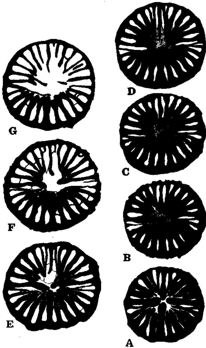
Abb. 6. Holotypus von Calophyllum (Groenlandophyllum) teichertii n. sp., Productus -Limestone Loc. T 67—101, zwischen River 13 und 14 (MMH 11928). 5 ×.
