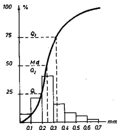
Abb. 2. Histogramm und Summenkurve der Korngrößen aus der Sandsteinbank der MFS 2.
