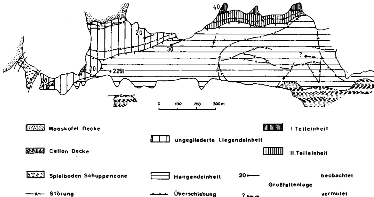
Abb. 8. Tektonische Karte des Elferspitz. Maßstab 1 : 10.000.
