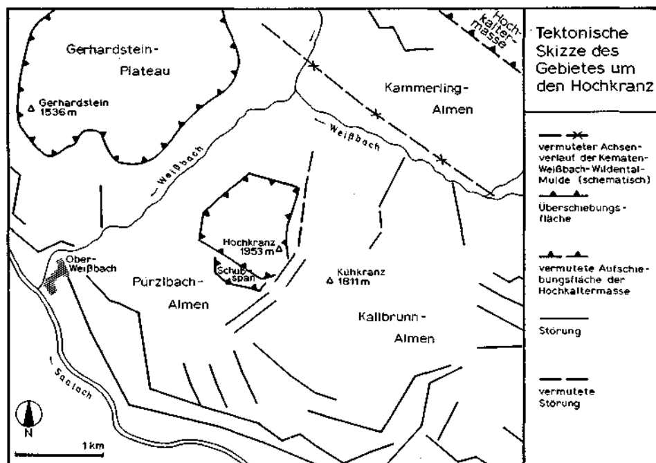
Abb. 2. Tektonische Skizze.
