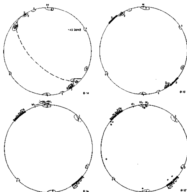
Diagramm 14. Zurückgekippte \beta -Maxima aller 3 Bereiche
