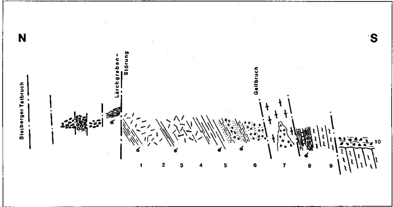
Abb. 1. Schematisches Nord-Süd-Profil durch den Nötschbach-Graben (Länge des Profils etwa 2,5 km) mit 1: Schiefer, Siltsteine und Kalke am Güterweg Hermsberg; 2: Diabas I; 3: Zwischenschiefer; 4: Diabas II; 5: Obere Schiefer; 6: Äquivalente der Erlachgraben-Gruppe; 7: Granitzug von Nötsch; 8: Graphitschiefer und Kalke des Unterdevons; 9: Phyllite und Quarzphyllite des Gailtal-Kristallins; 10: Gröden Sandsteine und Konglomerate.
