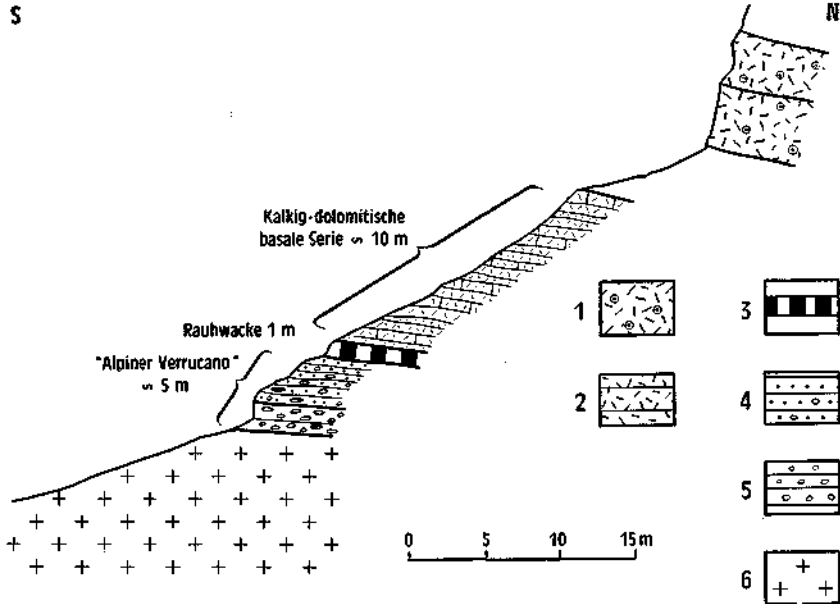
Abb. 3. Profil der Serie A bei der Kaserstatt-Alm in 1900 m Höhe.
