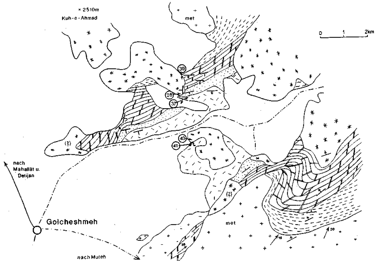
Abb. 2 a. Geologische Skizze der Gegend nördlich von Muteh. Grundlage: THIELE et al., 1968, Ergänzungen und Korrekturen THIELE, 1973.
