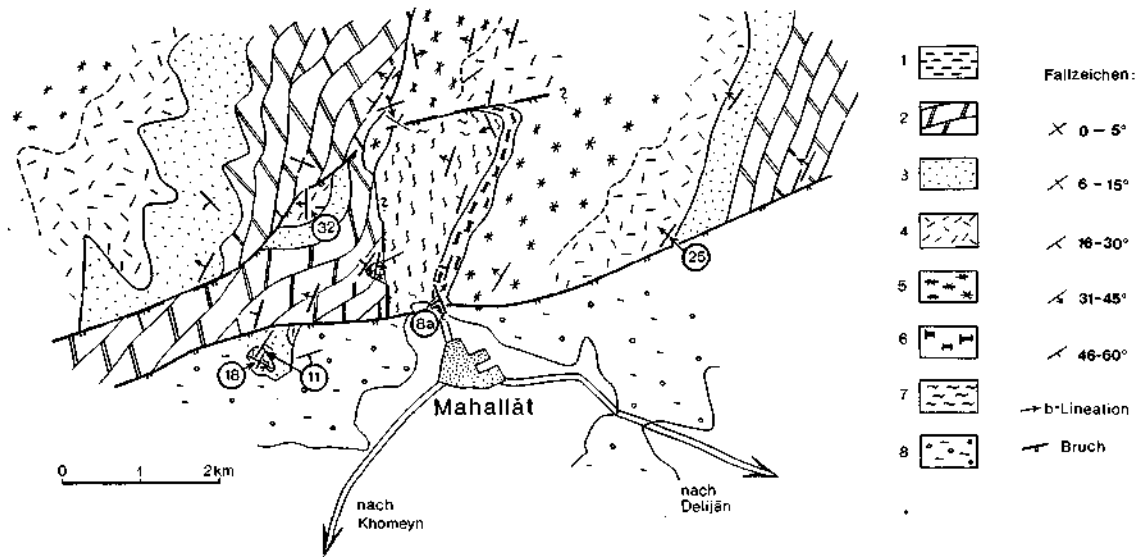
Abb. 2 b. Geologische Skizze der Umgebung von Mahallat.
