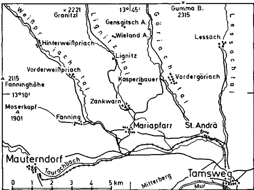
Abb. 1. Lage des untersuchten Vorkommens N Zankwam im Lungau/Salzburg.
