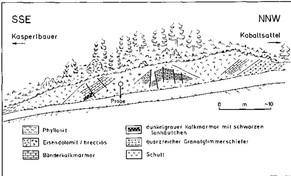
Abb. 3. Detailskizze des Karbonatgesteins-Aufschlusses am Zankwarner Berg.
