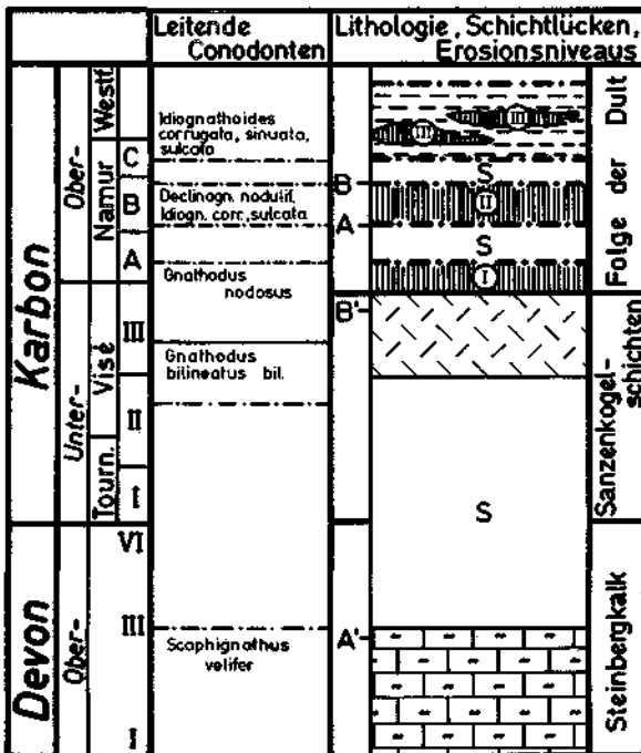
Abb. 3: Das Karbon des untersuchten Gebietes. Schematische, nicht maßstabgetreue Darstellung aller nachgewiesener Schichtglieder und Schichtlücken (S). Gesteinssignaturen wie auf Abb. 2. Durch A und B wird der Zeitpunkt der Erosionsniveaus markiert. A' und B' deutet das tiefste, nachgewiesene Eingreifen jedes Niveaus in der Karbonunterlage der Folge der Dult an.
