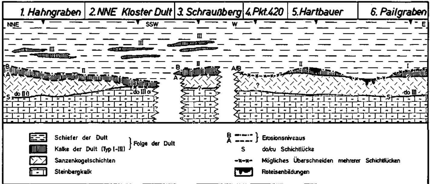
Abb. 2: Schematische Darstellung der Karbonablagerungen im Gebiet Hahngraben — Dult — Pailgraben. Entfernungs- und Mächtigkeitsverhältnisse der dargestellten Profile entsprechen nicht den natürlichen Gegebenheiten.
