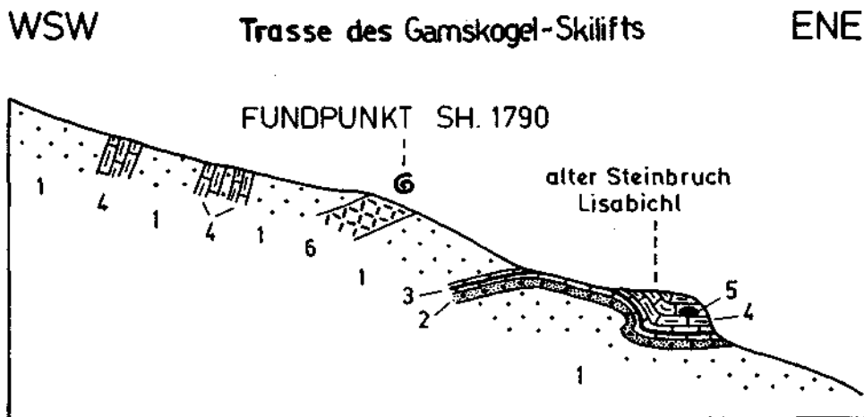
Abb. 2: Profil durch den Lisabichl. Aufgenommen von A. NOWOTNY. Signaturen wie bei Abb. 1.
