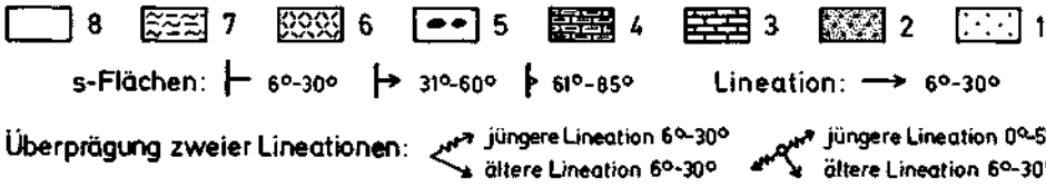
Abb. 1: Geologische Kartenskizze des Lisabichls, Aufgenommen von A. NOWOTNY. Erläuterung der Signaturen: 1 — Quarzphyllit und Quarzphyllonit. 2 — Graphitquarzit. 3 — Glimmerkalkmarmor. 4 — Bänderkalkmarmor. 5 — Graphitkalk. 6 — Eisendolomit. 7 — Kalkglimmerschiefer (Bündnerschiefer) der Tauernschieferhülle. 8 — Moräne, Gehängeschutt und Alluvionen.
