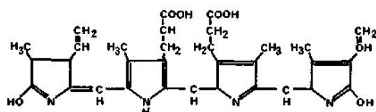
Abb. 3: Strukturformel von Biliverdin
