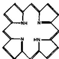
Abb. 4: Strukturformel von Porphyrin; 4 Pyrrol-Ringe durch 4 CH-Gruppen zu einem Ring verknüpft (vgl. KENNEDY & VEVERS: 1956)
