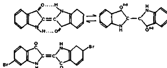
Abb. 5: Strukturformel indigoide Farbstoffe; a) Indigoblau (wasserunlöslich), b) Indigo-weiß (wasserlöslich), c) (6,6) Dibromindigo (Purpur). Für 1 g Purpur benötigt man 8000 Exemplare von Trunculariopsis trunculus (LINNÉ) oder 30.000 von Murex ( Bolinus ) brandaris LINNÉ oder gar 40.000 von Ocenebra ( Ocenebra ) erinacea (LINNÉ)
