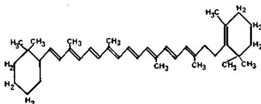
Abb. 2: Strukturformel von \beta -Carotin
