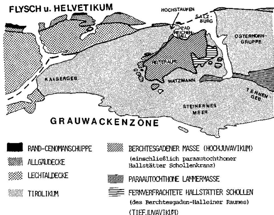
Abb. 1: Tektonische Übersichtsskizze des NW-Randes des tirolischen Bogens zwischen Inntal und Salzachtal
