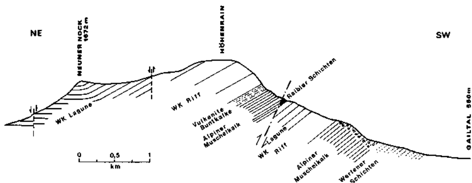
Abb. 5: NE-SW-Profil Bleibergertal – Gailltal. (Die horizontale Lage der Schichten im NE ergibt sich nur scheinbar, nämlich durch den Schnitteffekt: NE-Fallen der s-Flächen).
