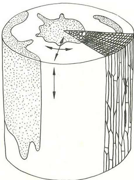
Abb. 1 Schema der Wegsamkeit des Fluorits in verkieselten Hölzern. Bevorzugung der durch Pflanzenstrukturen vorgegebenen Richtungen.
