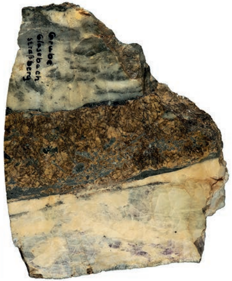
Abb. 18: Fluorit, Siderit, angeschliffen, Straßberg/Harz, Grube Glasebach, Inv.-Nr. 19/166
