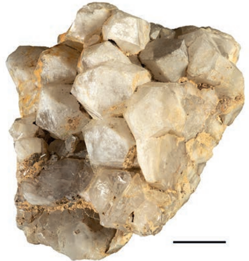
Abb. 12: Quarz xx ; Schneeberg/Erzgebirge, Inv.-Nr. 19/105
