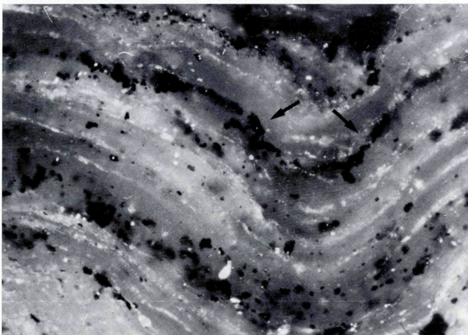
Abb. 4: Polierter Anschliff aus dem Vorkommen Tschingl. Größe des Bildausschnittes 2,4 \times 1,6 mm. Nicols gekreuzt. Die rhythmische Wechsellagerung von lichtgrauen quarzitischen, weiß-grauen bis grauweißen Rutil- und Glimmerreichen, sowie grauschwarzen (unter der Präparatoberfläche liegend) bis schwarzen Erzlagen ist auf dieser Abbildung gut zu erkennen. Ebenso kommt eine Fältelung des gesamten Stoffbestandes deutlich zur Geltung. Daß die Durchbewegung ein postkristallines Ereignis ist, belegt auch die gestaltliche Einregelung (Pfeil) der Erzkörner.
