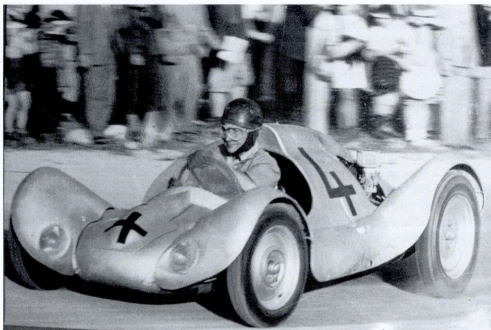
Abb. 8: Der Eigenbau – Mittelmotor – Rennwagen feierte in der Wiener Krieau 1953 seine Premiere – hier in Sandbahnausrüstung.
