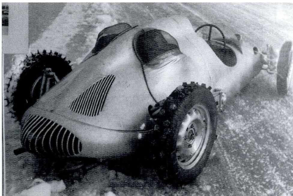
Abb. 7: Eigenbau – Mittelmotor – Rennwagen aus dem Jahre 1952, hier bestückt mit speziellen Spikes-Reifen für Eisrennen.
