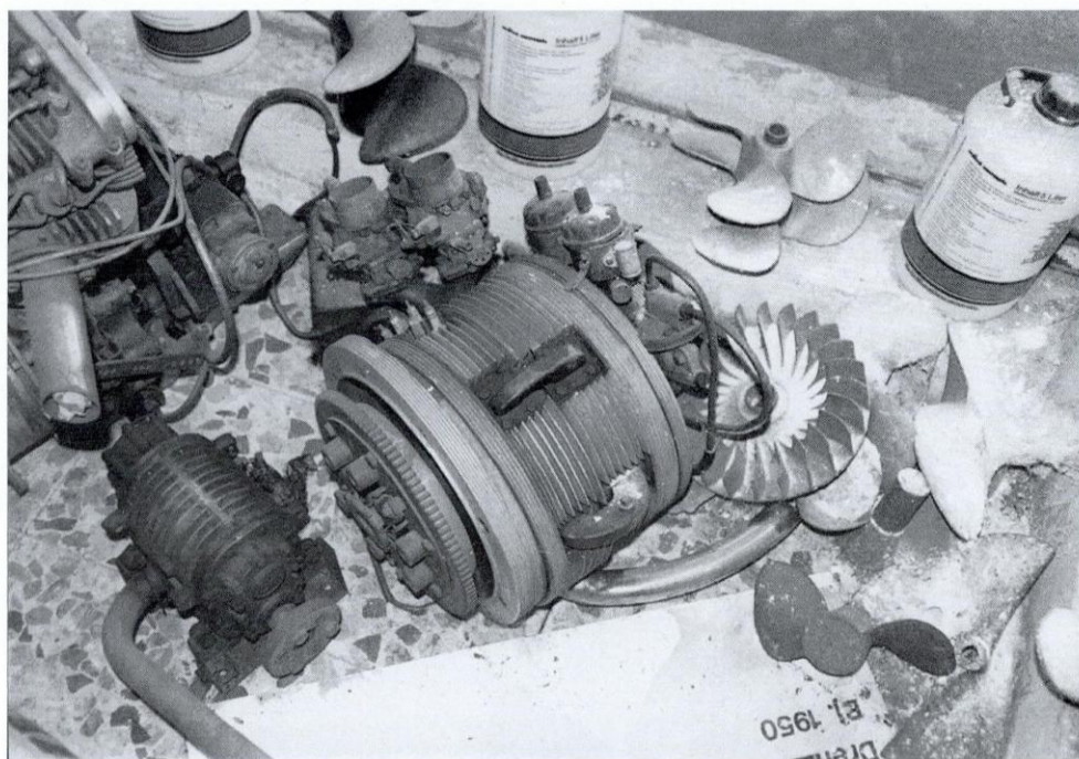
Abb. 21: Der Drehkolbenmotor von Otto Mathé.
