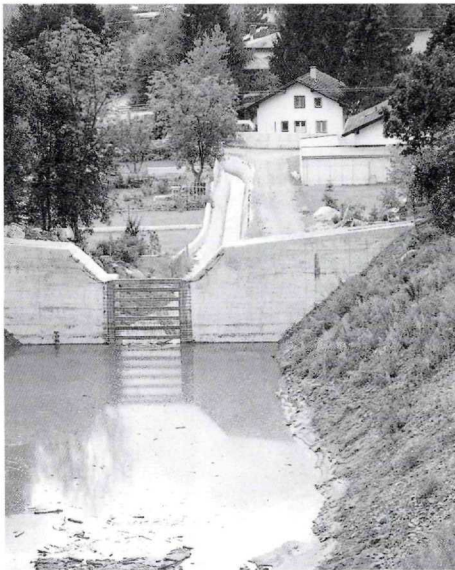
Abb. 11. Geschiebedosiersperre oberhalb der WARTSCHEN-SIEDLUNG und WARTSCHEN-BACH-Verbauung am unteren Schwemmkegel, Verbaumaßnahmen 1986.
