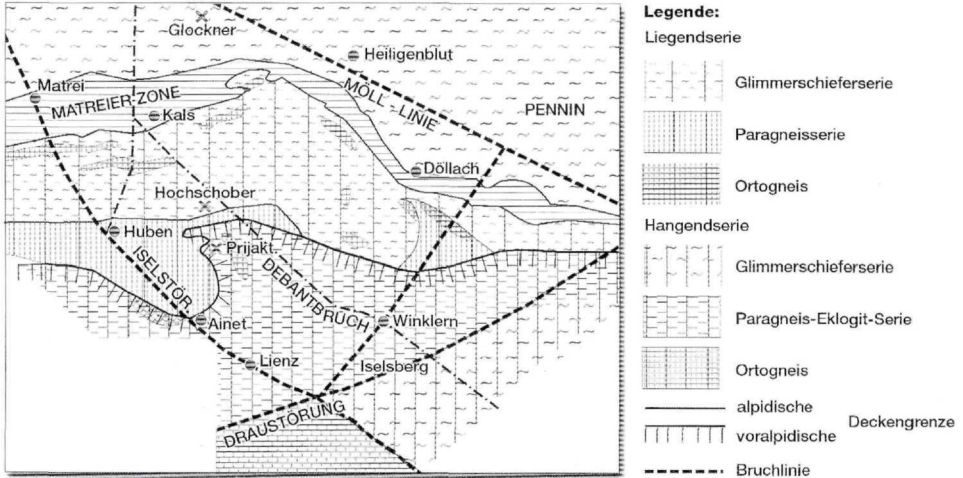
Skizze 1. Geologisch-tektonische Übersichtsskizze der SCHOBERGRUPPE (TOLLMANN, 1977)
