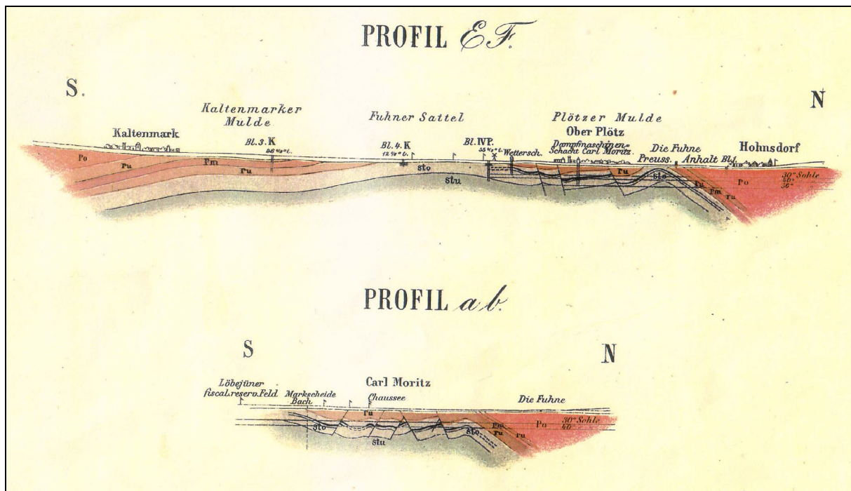
Abb. 3: Ausschnitt aus der geognostischen Darstellung des Steinkohlengebirges und Rotliegenden in der Gegend nördlich von Halle a. Saale von Dr. Hugo Laspeyres, Berlin 1870. Hier: Profil E F
