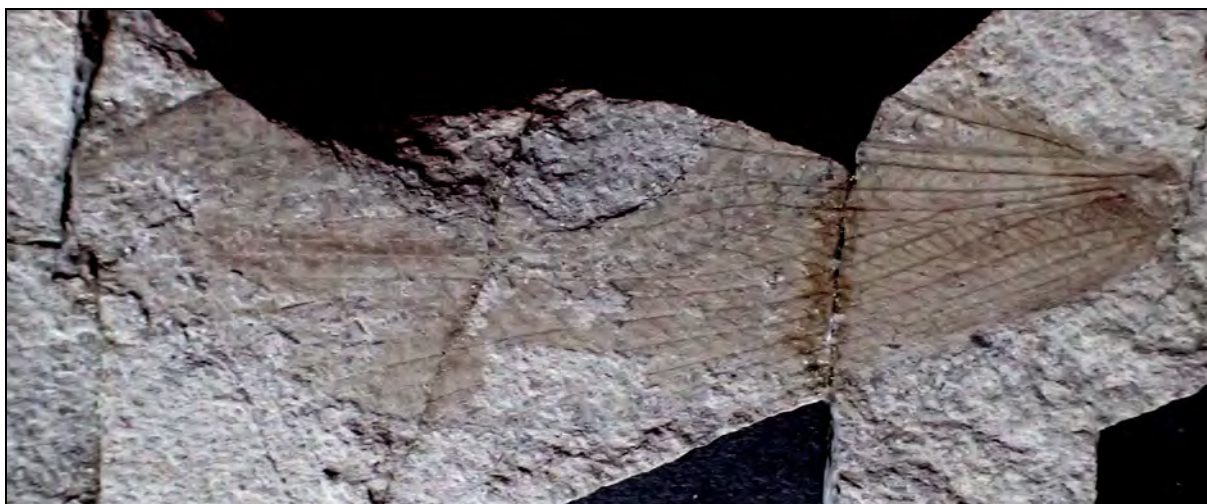
Abb. 5: Fanzus grandis n. gen. et n. sp., Gegendruck.
