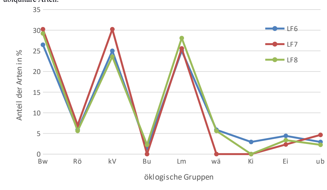
Abb. 9: Ökologisches Profil der Lepidopterenvergesellschaftung im Untersuchungsbereich LF6 bis LF8.
