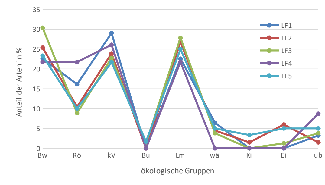
Abb. 8: Ökologisches Profil der Lepidopterenvergesellschaftung im Untersuchungsbereich LF1 bis LF5. Legende: Bw = Bruchwald-bewohnende Arten, Rö = Röhricht-bewohnende Arten, kV = Arten der krautigen Vegetation, Bu = Buchenwald-bewohnende Arten, Lm = Laubmischwald-bewohnende Arten, wä = wärmeliebende Arten, Ki = Arten der autochthonen Kiefernwälder, Ei = Arten der Eichengehölze, ub = ubiquitäre Arten.
