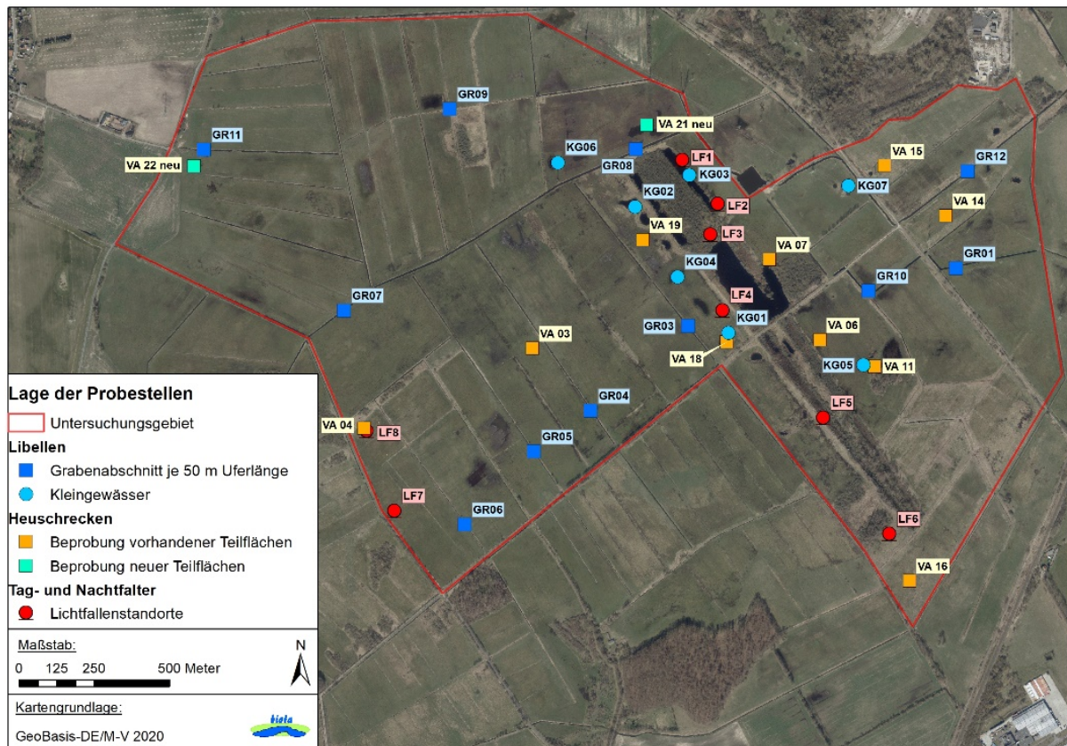
Abb. 5: Lage der Probestellen der untersuchten Artengruppen.
