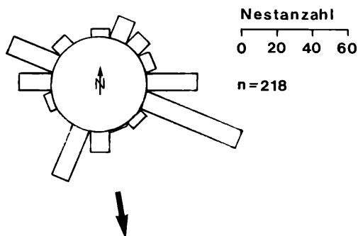
Abb. 4: Mehlschwalben-Nester (1980 bis 1983) an beiderseits bzw. allseits gleichwertigen Häusern ( \alpha = 169,6^\circ ; a = 0,215 ; p < 0,01 ).
