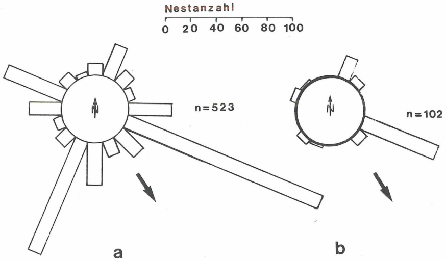
Abb. 1: a: Exposition der Nester in Horitschon (links, = a) und in Haschendorf (rechts, = b). Pfeil = errechnete Vorzugsrichtung. a: \alpha = 146,8^\circ ; a = 0,348 ; p < 0,001 . b: \alpha = 146,9^\circ ; a = 0,652 ; p < 0,001 .
