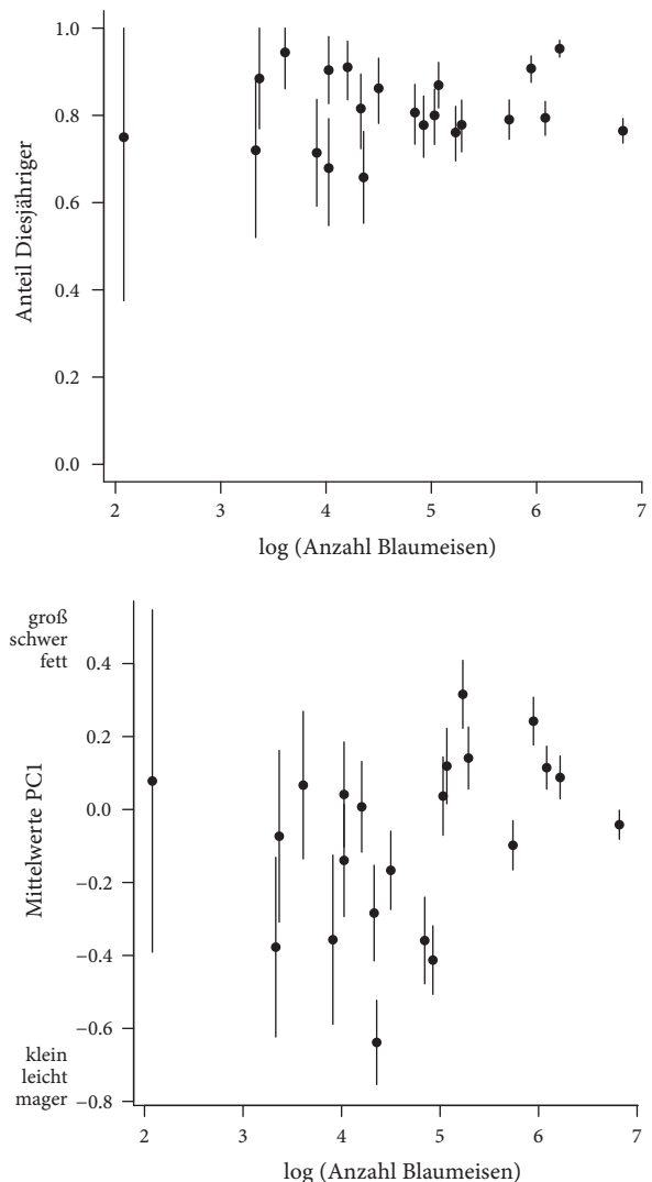
Abb. 4: Zusammenhang zwischen dem Anteil Diesjähriger (oben) und dem Mittelwert der ersten Hauptkomponente (PC1, Maß für die Körpergröße, unten) pro Jahr und der Anzahl Durchzügler (log-transformiert) für die Blaumeise. Vertikale Linien zeigen für den Anteil Juveniler das Vertrauensintervall und für PC1 die Standardfehler an. – Blue Tit: Correlation between the proportion juveniles (above) and the mean of PC1 („Mittelwerte PC1“, mass for large body size and high fat reserves, see Tab. 4) per year and the number of migrants caught (log-transformed). Vertical lines indicate 95 % confidence intervals for the proportion of juveniles and standard errors for the mean of PC1.
