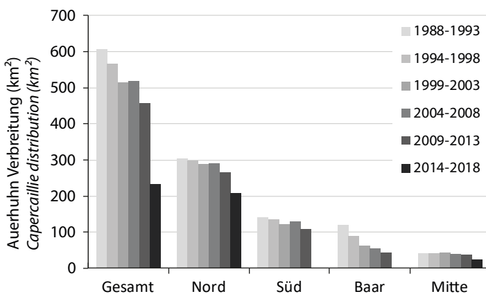
Abb. 5: Die Fläche der Auerhuhn-Verbreitung (in km 2 ) im Schwarzwald (gesamt) und nach Teilgebieten, aufgeteilt auf die Kartierungszeiträume (s. Abb. 1). – Capercaillie distribution (in km 2 ) shown for the Black Forest (Gesamt) and the different sub areas of the Black Forest per time period.
