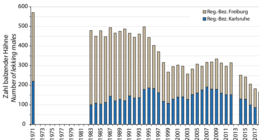
Abb. 2: Die Zahl balzender Hähne pro Jahr, die im Schwarzwald erfasst wurden. Die erste zuverlässige Zählung von 1971 ist als Vergleich dargestellt (Roth 1974). Die Daten wurden von der Auerwildhegengemeinschaft im Regierungsbezirk Freiburg und den Auerwildhegeringen Freudenstadt und Calw erhoben und von der FVA zusammengetragen. – Number of capercaillie males counted at leking sites in the Black Forest per year, shown for the administrative regions "Freiburg" and "Karlsruhe". The result of the first systematic census of 1971 is presented as a reference (Roth 1974), since 1983 capercaillie males have been counted yearly. The census is organized by the hunter's associations: "Auerwildhegengemeinschaft", "Auerwildhegering Freudenstadt" and "Auerwildhegering Calw".
