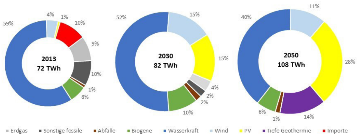
Abb.11: Zusammensetzung der Aufbringung von Elektrizität
