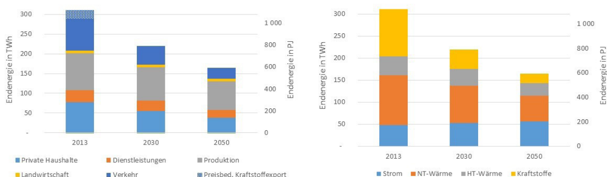
Abb.5: Gliederung des Endenergiebedarfs nach Sektoren (links) und Nutzenergiekategorien (rechts)
