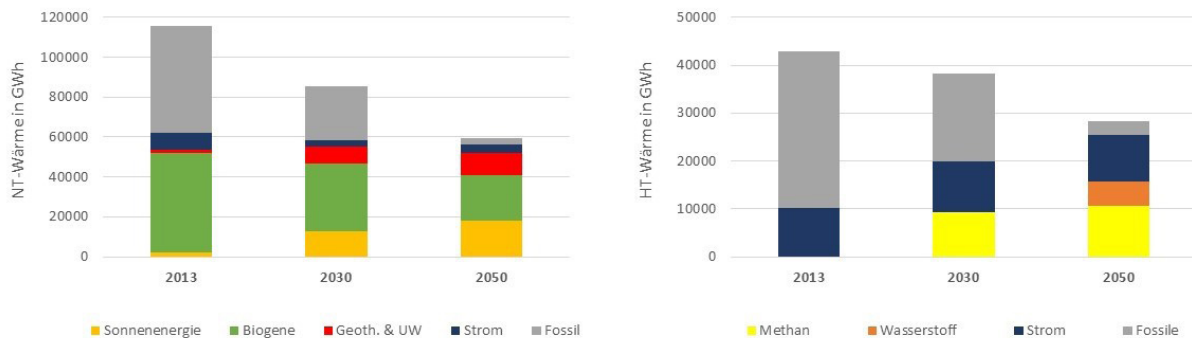
Abb.8: Aufbringung der Niedertemperaturwärme (links) und Hochtemperaturwärme (rechts)
