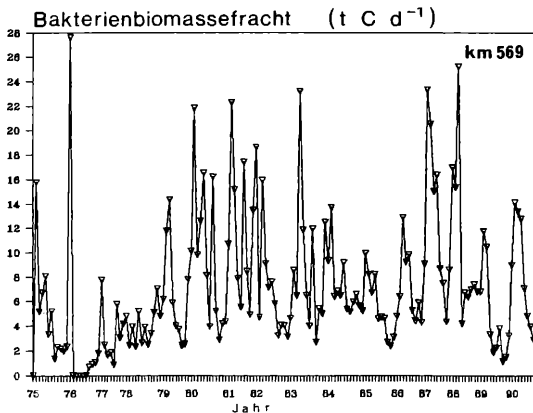
Abb. 4: Bakterienbiomassefracht ( \text{t C d}^{-1} ) in der Elbe bei Lauenburg (Hochrechnung)
