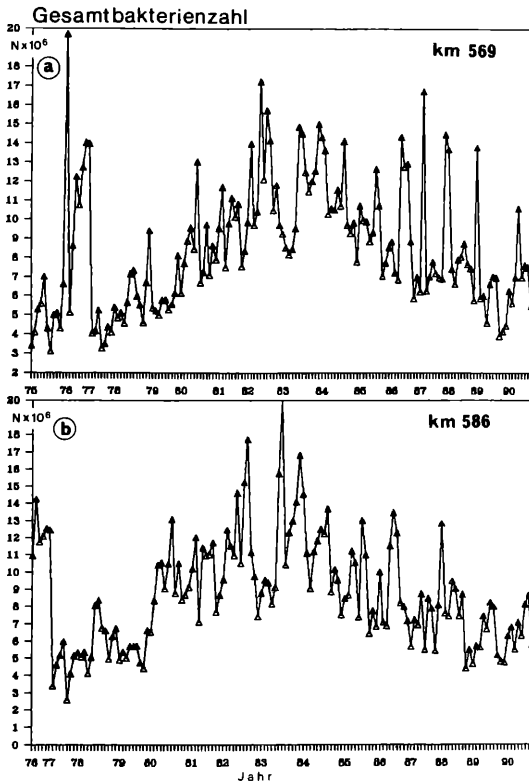
Abb. 2: Gesamtbakterienzahlen (Zellen \text{ml}^{-1} ) a Lauenburg b Geesthacht
