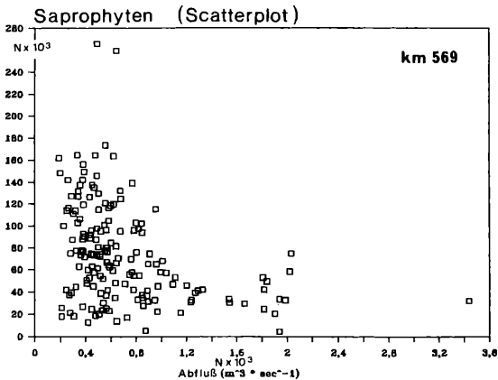
Abb. 11: Scatterplot für Koloniezahlen auf Hefeextrakt-Pepton-Agar nach 14 Tagen Bebrütung und Abfluß
