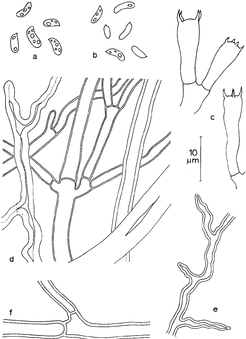
Abb. 2. Antrodiella onychooides . a, b Sporen, c Basidie, d Hyphen aus der Trama, mit zwei dünnwandigen generativen Hyphen, mit einer dickwandigen und einer vollen Skeletthyphie und mit einer verzweigten sklerifizierten Hyphe, e verzweigte sklerifizierte Hyphe, f dickwandigere generative Hyphe, Vergr. 2000 x.
