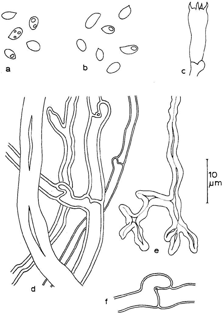
Abb. 1. Antrodiella semisupina . a, b Sporen, c Basidie, d Hyphen aus der Trama, mit einer dünn- und einer dickwandigen generativen Hyphe sowie einer vollen und einer dickwandigen Skeletthyphye, e stark verzweigte sklerifizierte Hyphye, f generative Hyphye mit großer Schnalle. Vergr. 2000 x.
