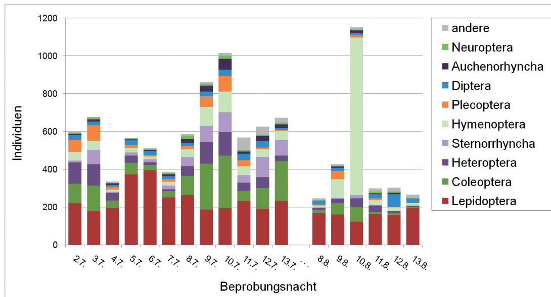
Abb. 11: Angelockte Insekten/Beprobungsnacht.
